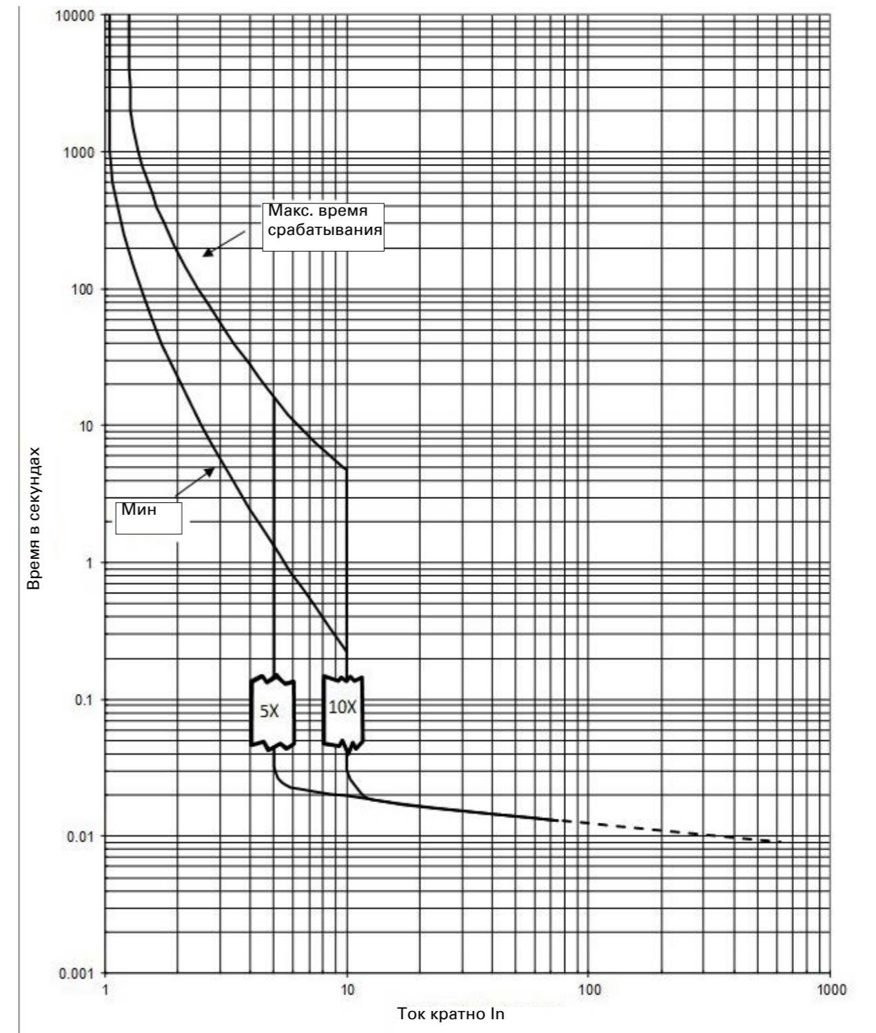
Защита системы и линии с PDE2 TMTU; 160 A, 200 A и 250 A при 240 В, 415 В и 440 В
