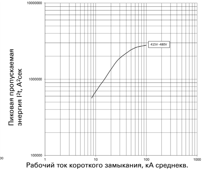
Пропускаемая энергия I 2 t; PDE9 ETU PXR10 LI; 63 А и 100 А при 415 В и 440 В
