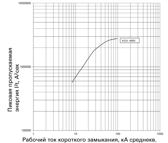
Пропускаемая энергия I^2t ; PDE2 TMTU; 160 А при 415 В и 440 В
