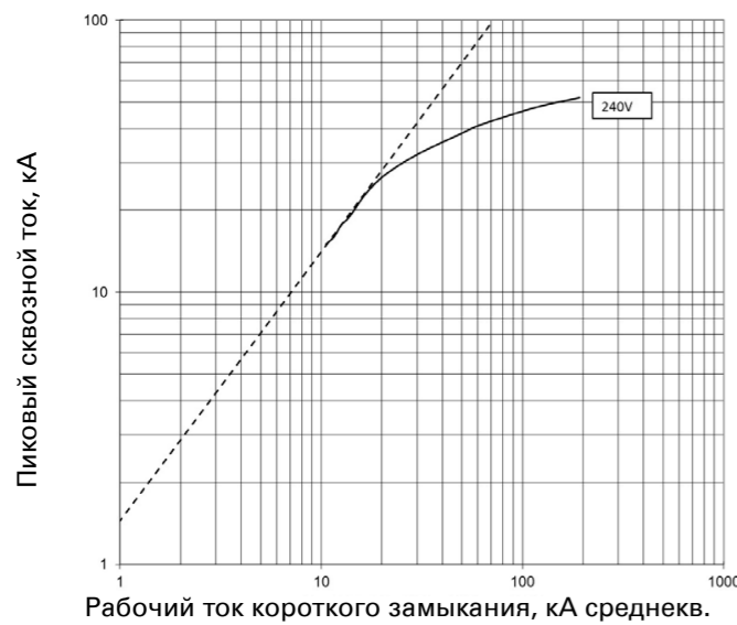
Сквозной ток I_D ; PDE3 TMTU; 500 А и 630 А при 240 В
