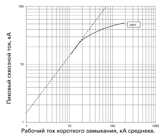
Сквозной ток I_D ; PDE3 ETU PXR10 LI; 630 А при 240 В
