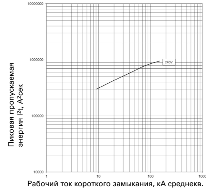
Пропускаемая энергия I^2t ; PDE2 TMTU; 160 А при 240 В
