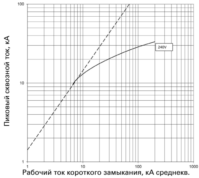
Сквозной ток I_D PDE2 TMTU; 250 А при 240 В
