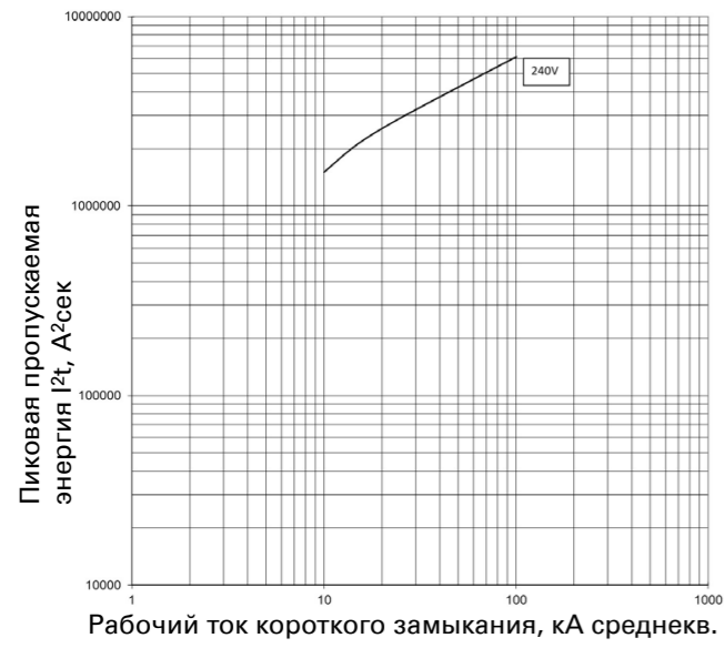
Пропускаемая энергия I^2t ; PDE4 TMTU; 800 А при 240 В
