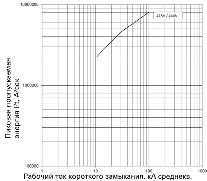
Пропускаемая энергия I 2 t; PDE3 TMTU; 500 А и 630 А при 415 В и 440 В
