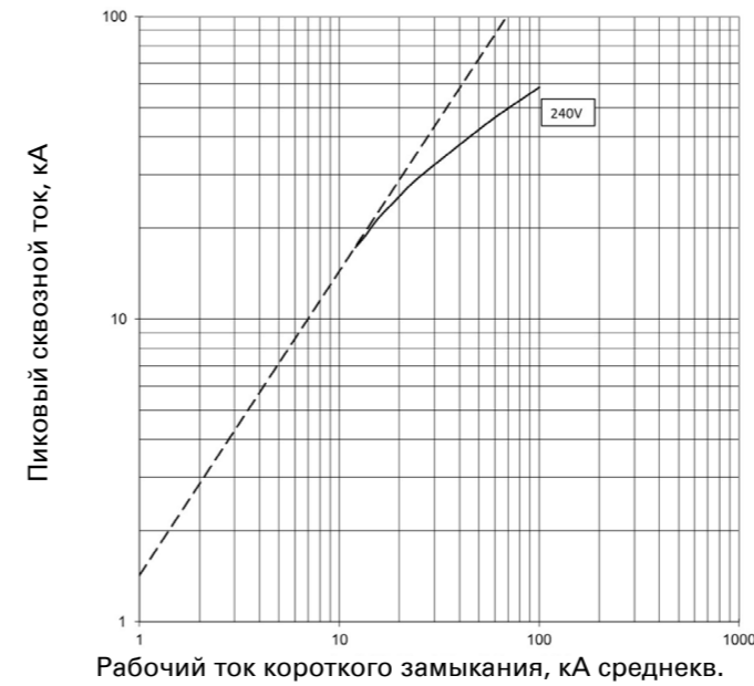
Рабочий ток короткого замыкания, кА среднев.
