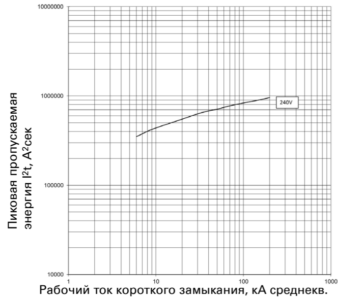
Пропускаемая энергия I 2 t; PDE2 TMTU; 200 А при 240 В
