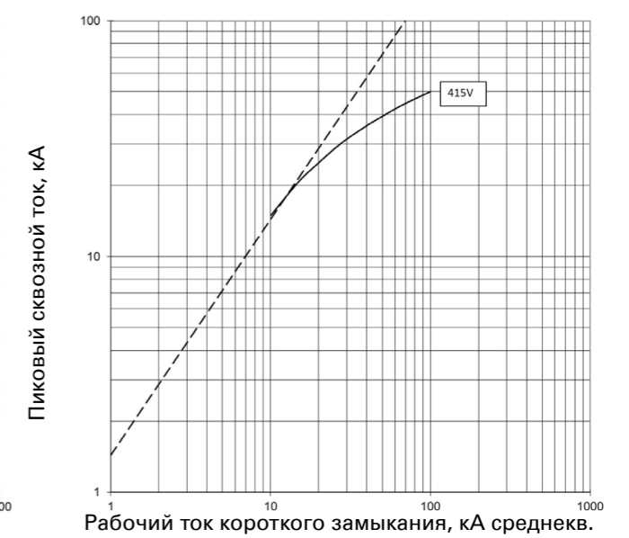
Сквозной ток I_D ; PDE3 ETU PXR10 LI; 400 А при 415 В и 440 В
