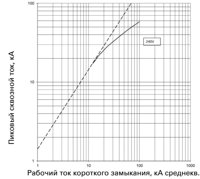
Рабочий ток короткого замыкания, кА среднев.
