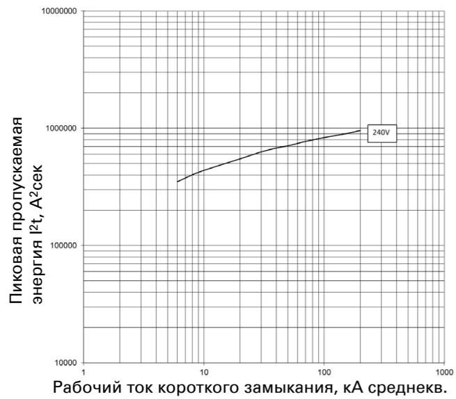
Пропускаемая энергия I 2 t; PDE2 TMTU; 250 А при 240 В
