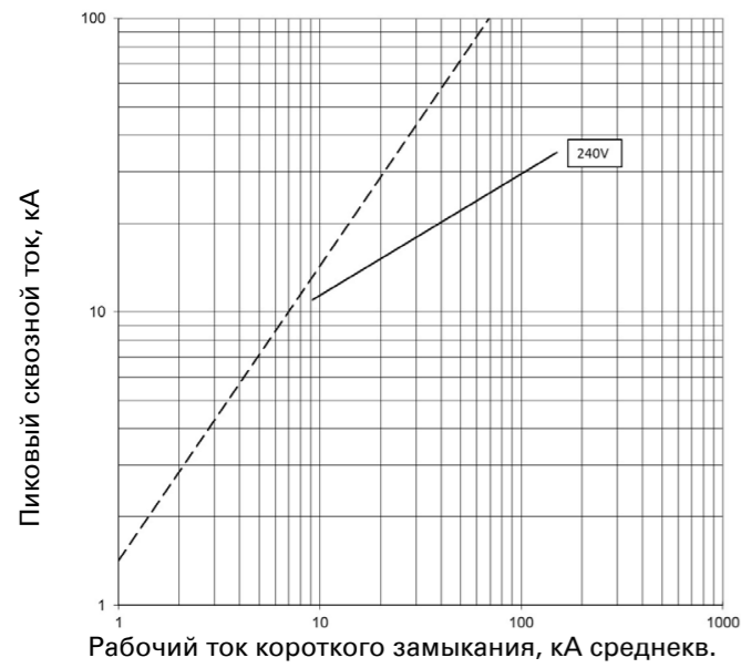
Сквозной ток I_D PDE2 ETU PXR10 LSI; 100 А и 160 А при 240 В
