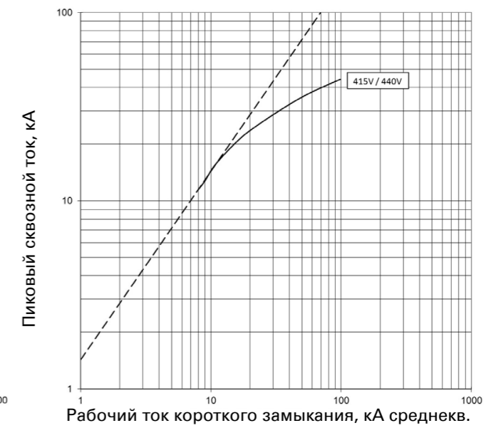
Сквозной ток I_D PDE2 ETU PXR10 LI; 250 А при 415 В и 440 В
