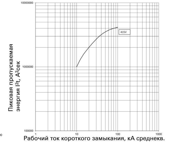
Пропускаемая энергия I 2 t; PDE3 ETU PXR10 LI; 400 А при 415 В
