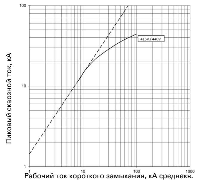
Сквозной ток I_D PDE2 ETU PXR10 LSI; 250 А при 415 В и 440 В
