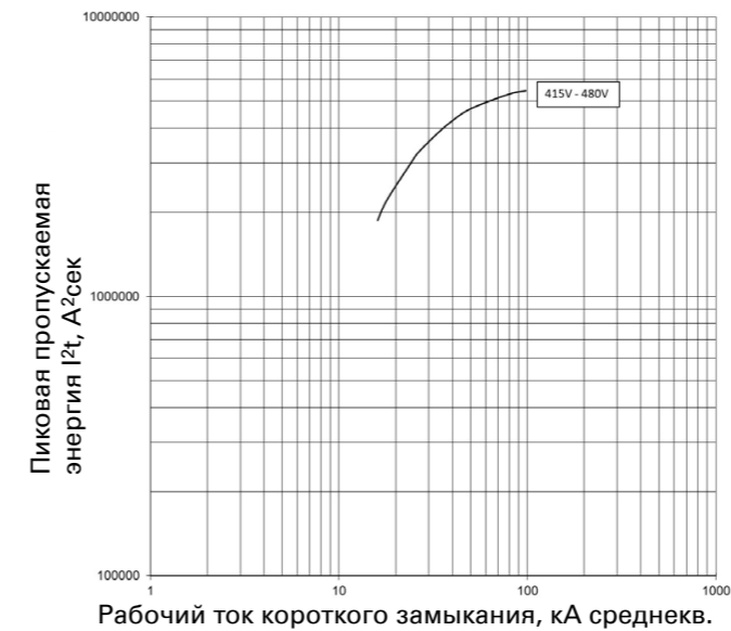
Пропускаемая энергия I 2 t; PDE3 ETU PXR10 LI; 400 А при 440 В
