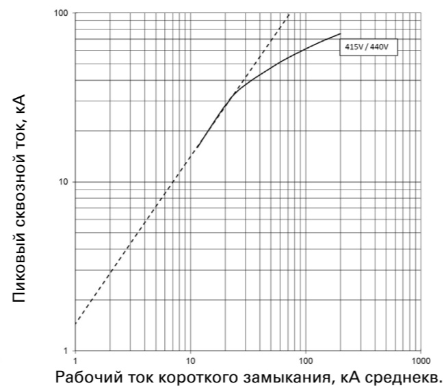
Сквозной ток I_D ; PDE3 TMTU; 500 А и 630 А при 415 В и 440 В
