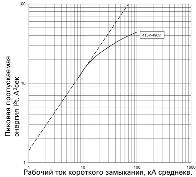
Пропускаемая энергия I 2 t; PDE2 TMTU; 200 А при 415 В и 440 В
