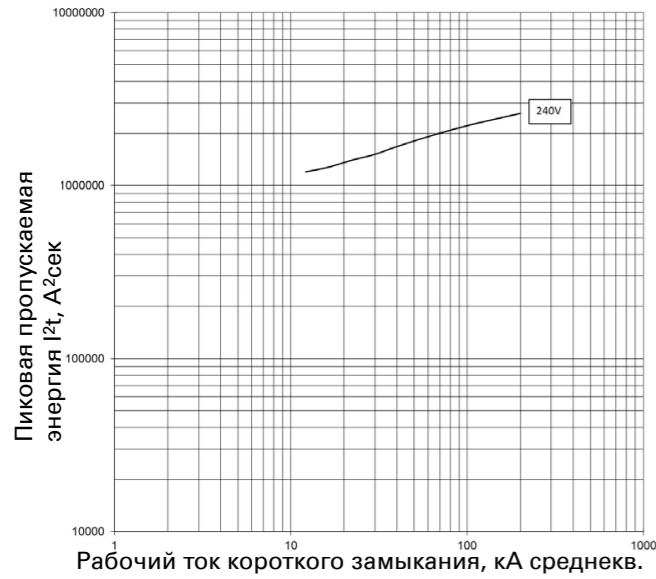
Пропускаемая энергия I 2 t; PDE3 TMTU; 250, 320, 400 А при 240 В
