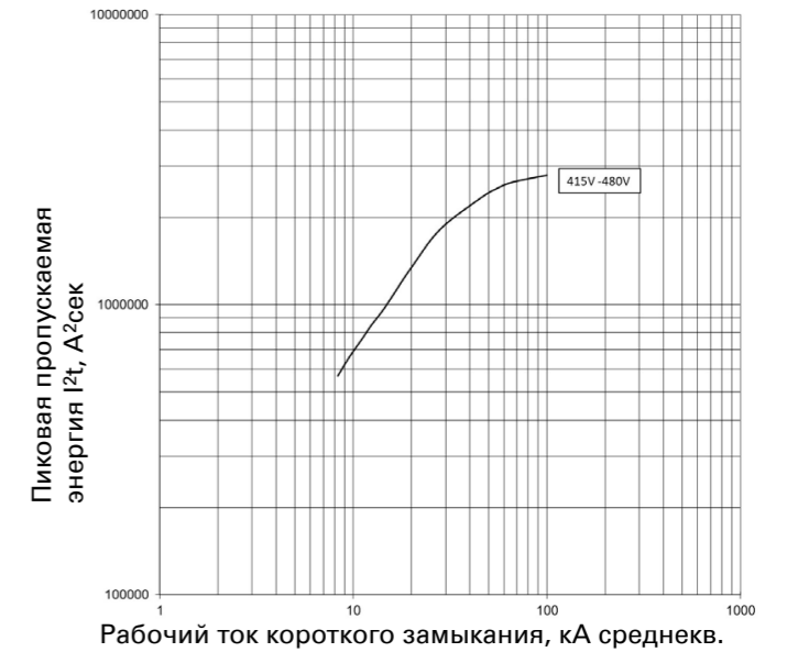
Пропускаемая энергия I 2 t; PDE2 ETU PXR10 LI; 160 А при 415 В и 440 В
