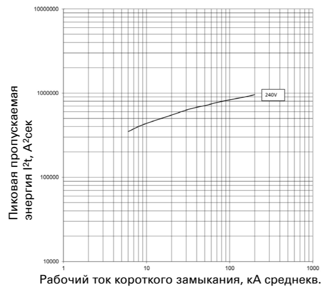
Пропускаемая энергия I 2 t; PDE2 ETU PXR10 LSI; 220 А при 240 В
