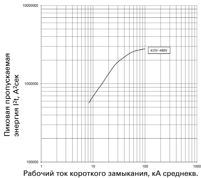
Пропускаемая энергия I 2 t; PDE2 ETU PXR10 LSI; 100 А и 160 А при 415 В и 440 В
