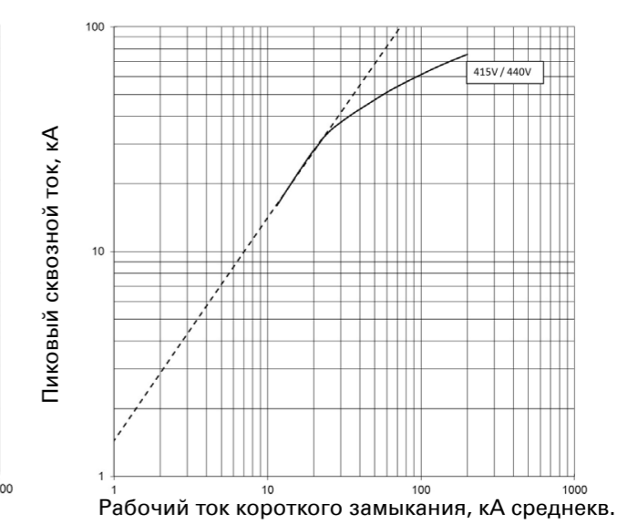
Сквозной ток I_D ; PDE3 ETU PXR10 LI; 630 А при 415 В и 440 В
