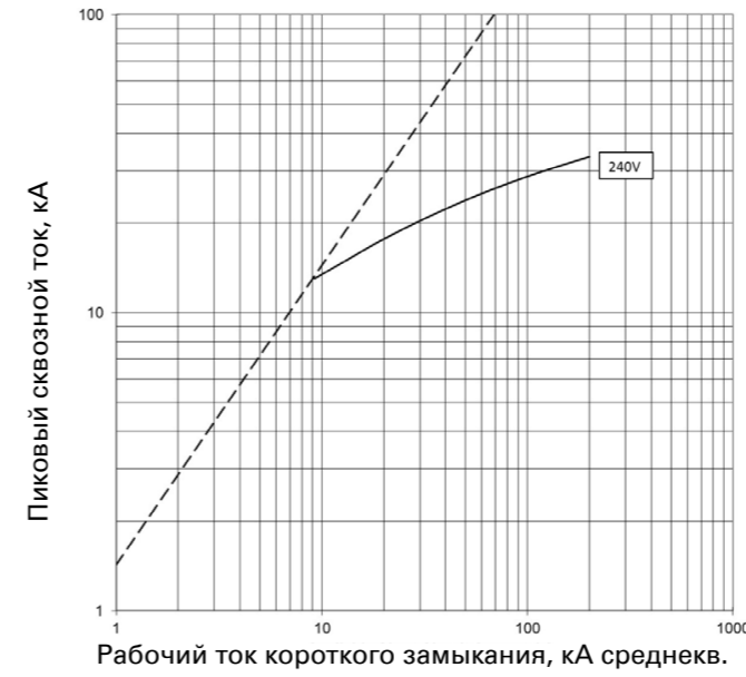
Сквозной ток I_D PDE2 ETU PXR10 LI; 200 А при 240 В
