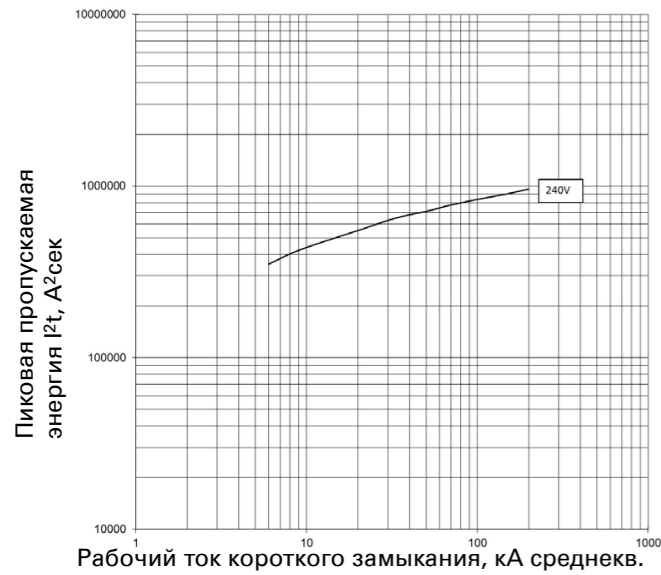
Пропускаемая энергия I 2 t; PDE2 ETU PXR10 LI; 250 А при 240 В
