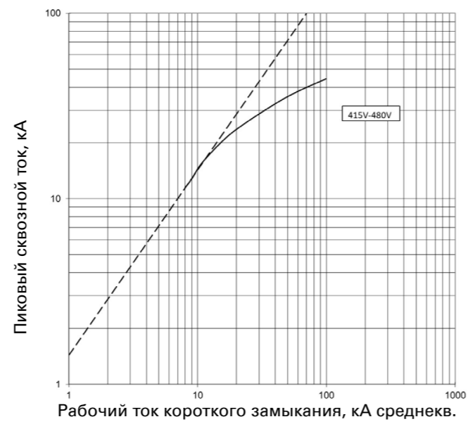
Сквозной ток I_D PDE2 ETU PXR10 LSI; 100 А и 160 А при 415 В и 440 В
