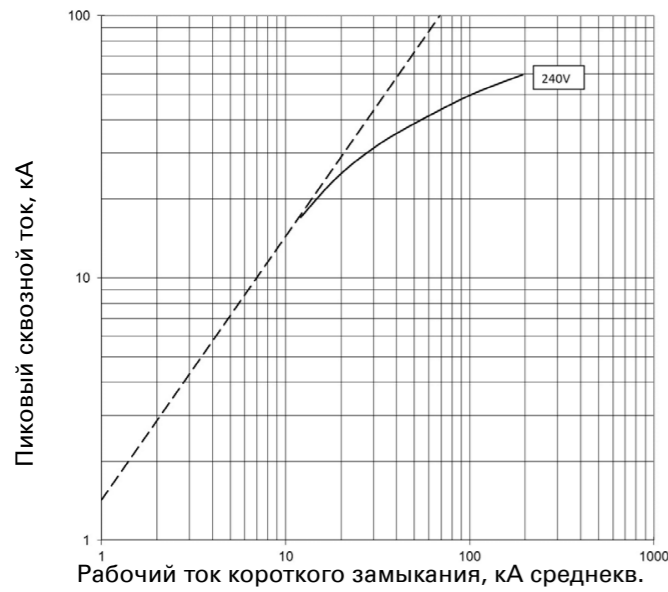
Сквозной ток I_D ; PDE3 TMTU; 250, 320, 400 А при 240 В
