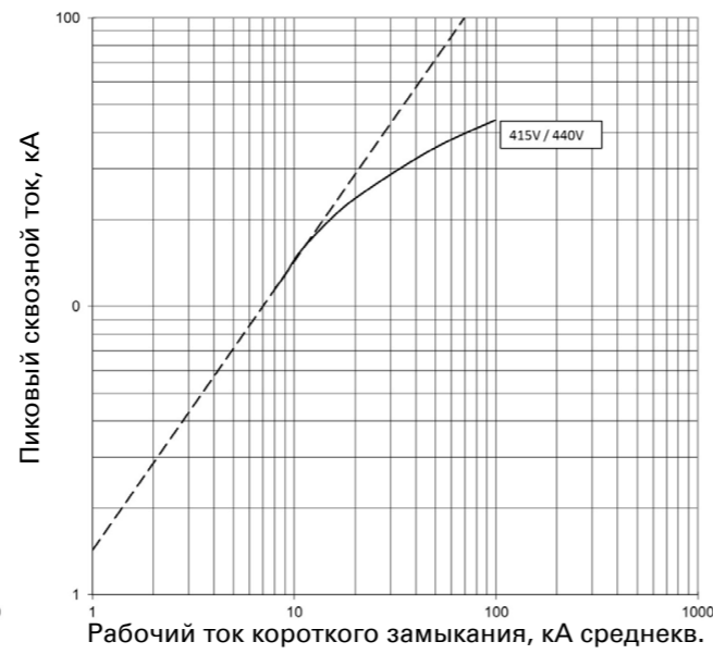
Сквозной ток I_D PDE2 TMTU; 250 А при 415 В и 440 В
