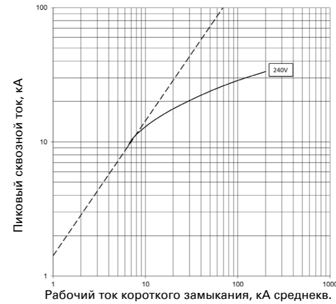
Сквозной ток I_D PDE2 ETU PXR10 LI; 250 А при 240 В
