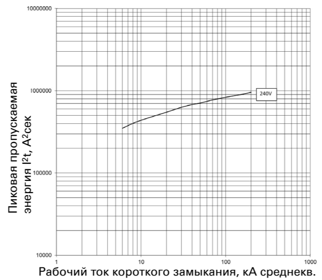
Пропускаемая энергия I 2 t; PDE2 TMTU; 250 А при 415 В и 440 В
