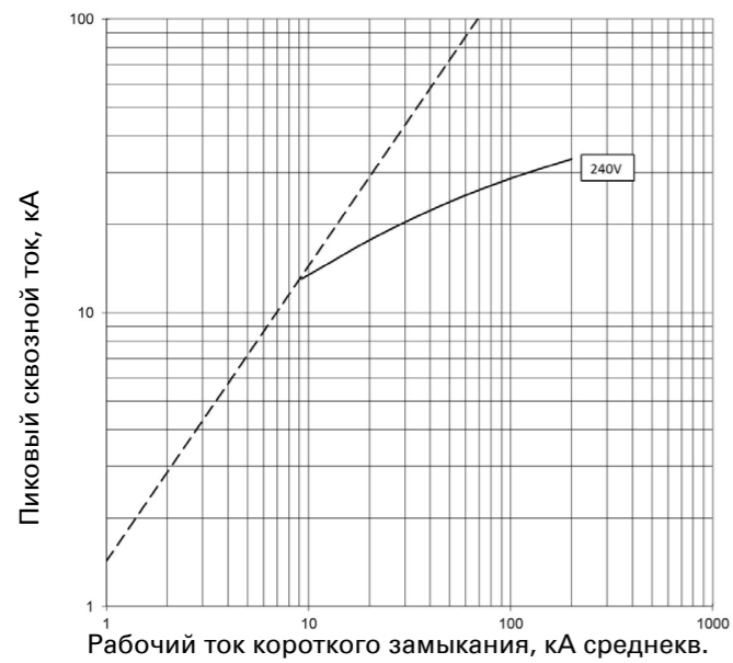
Сквозной ток I_D PDE2 ETU PXR10 LSI; 250 А при 240 В
