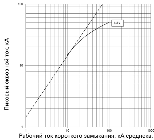
Сквозной ток I_D ; PDE3 TMTU; 250, 320, 400 А при 415 В и 440 В
