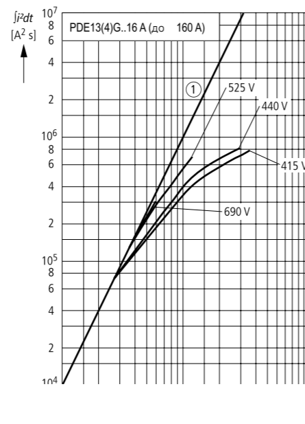
Пропускаемая энергия I^2t ; PDE1 TMTU PDE13(4)G..16 A (до 160 A)
