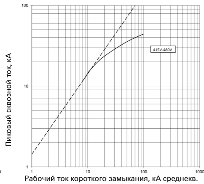
Сквозной ток I_D PDE2 ETU PXR10 LI; 160 А при 415 В и 440 В
