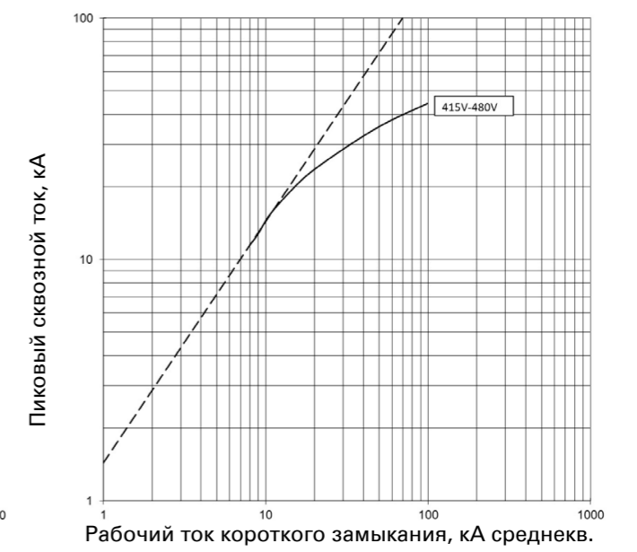
Сквозной ток I_D ; PDE9 ETU PXR10 LI; 63 А и 100 А при 415 В и 440 В
