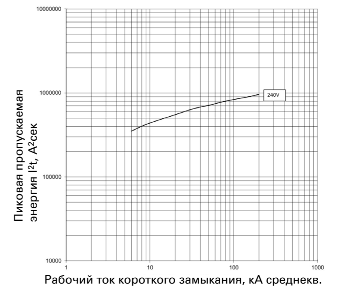
Пропускаемая энергия I 2 t; PDE2 ETU PXR10 LI; 200 А при 415 В и 440 В
