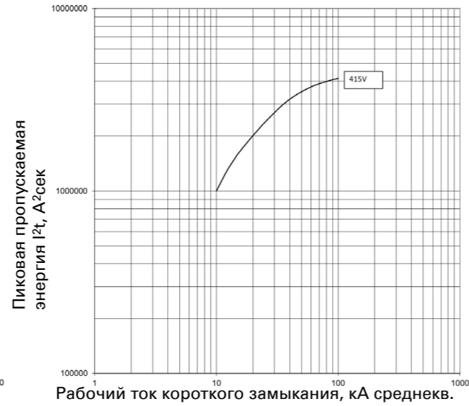
Пропускаемая энергия I 2 t; PDE3 TMTU; 250, 320, 400 А при 415 В и 440 В
