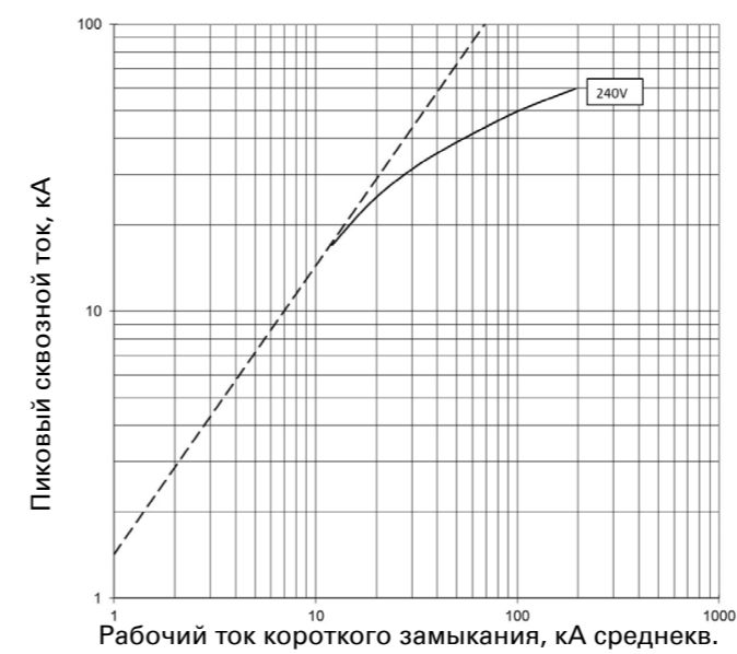
Сквозной ток I_D ; PDE3 ETU PXR10 LI; 400 А при 240 В
