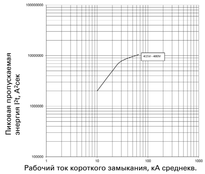
Пропускаемая энергия I^2t ; PDE4 PXR10 LI; 800 А при 415 В и 440 В
