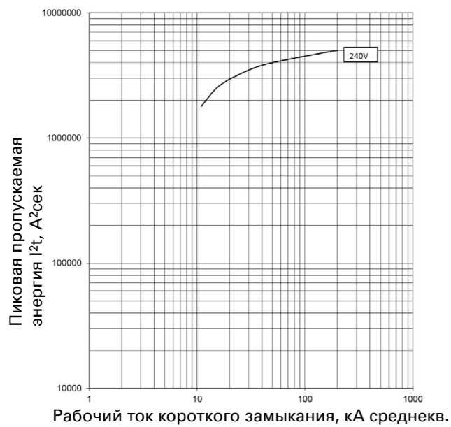
Пропускаемая энергия I 2 t; PDE3 TMTU; 500 А и 630 А при 240 В
