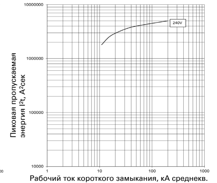
Пропускаемая энергия I 2 t; PDE3 ETU PXR10 LI; 630 А при 240 В
