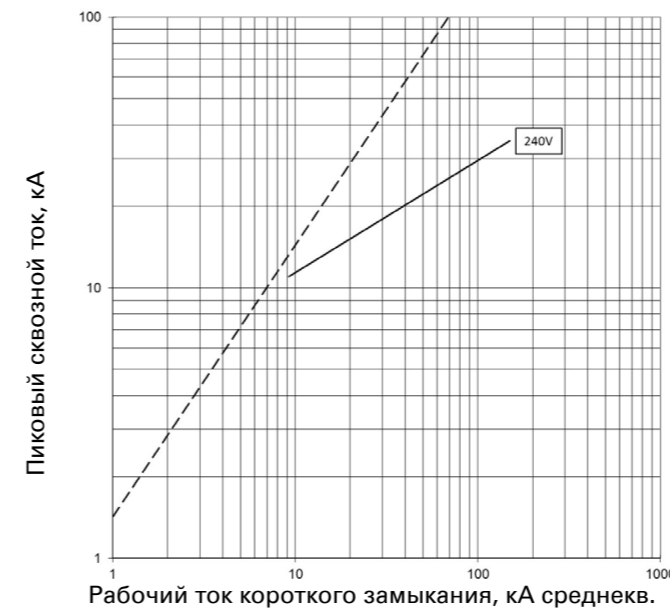
Сквозной ток I_D ; PDE9 ETU PXR10 LI; 63 А и 100 А при 240 В
