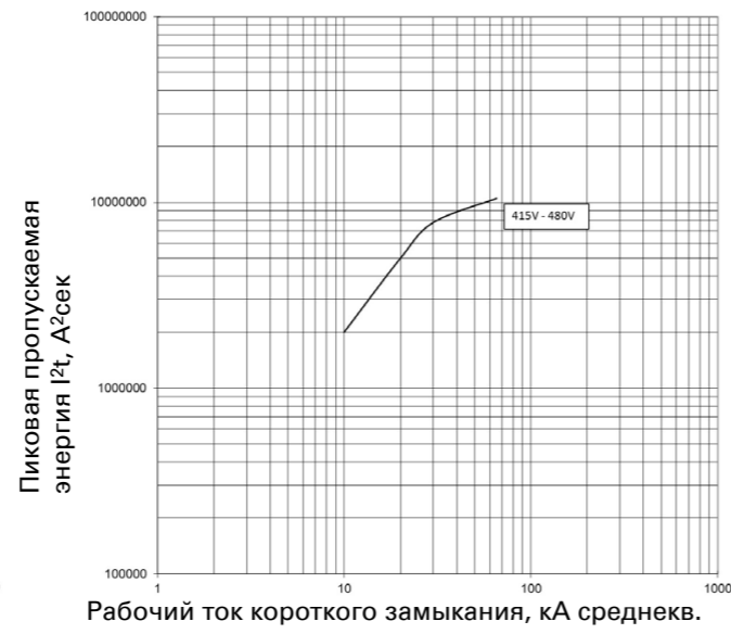
Пропускаемая энергия I^2t ; PDE4 TMTU; 800 А при 415 В и 440 В
