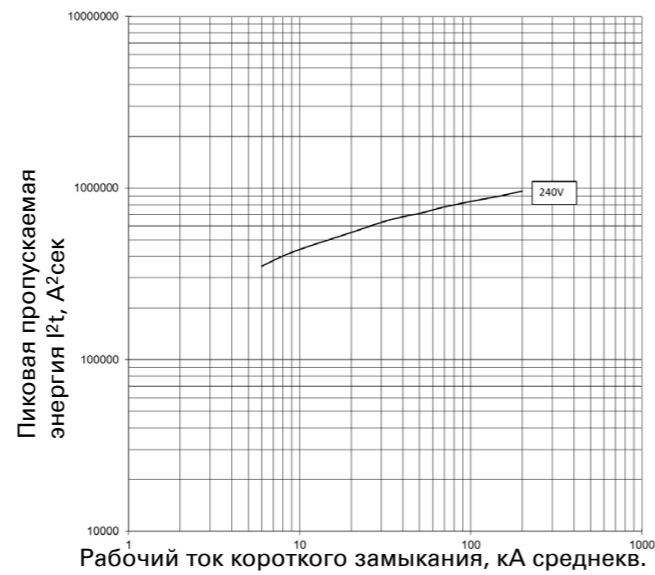
Пропускаемая энергия I 2 t; PDE2 ETU PXR10 LI; 250 А при 415 В и 440 В
