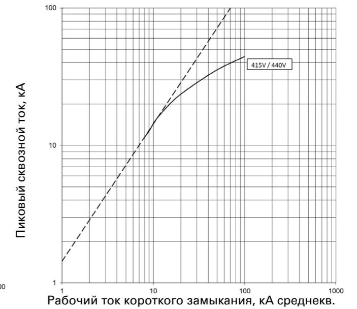
Сквозной ток I_D PDE2 ETU PXR10 LI; 200 А при 415 В и 440 В
