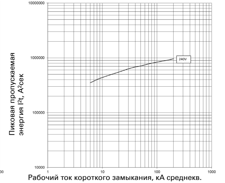
Пропускаемая энергия I 2 t; PDE2 ETU PXR10 LSI; 220 А при 415 В и 440 В
