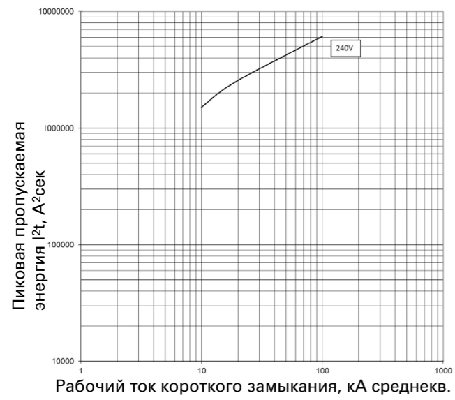
Пропускаемая энергия I^2t ; PDE4 PXR10 LI; 800 А при 240 В
